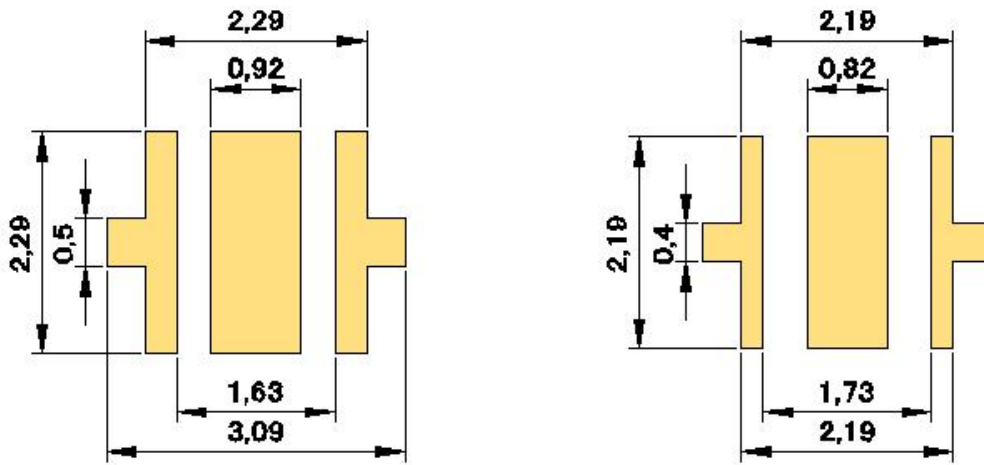
建议焊盘图
