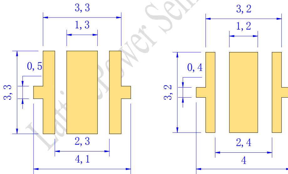
建议焊盘图
